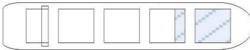
Рис.3.3.7.2 Варіанти навантаження внаслідок зледеніння для лісових палубних вантажів
