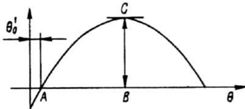
Рис. 1.3 Визначення перекидального моменту у неробочому стані
