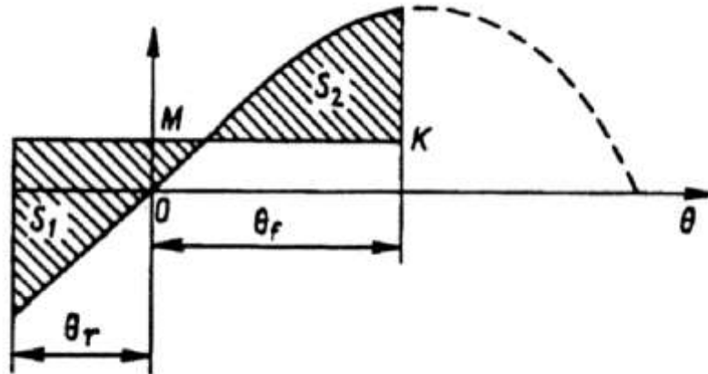
Рис. 2.1.2.2 Визначення перекидального моменту за діаграмою статичної остійності з урахуванням кута заливання
