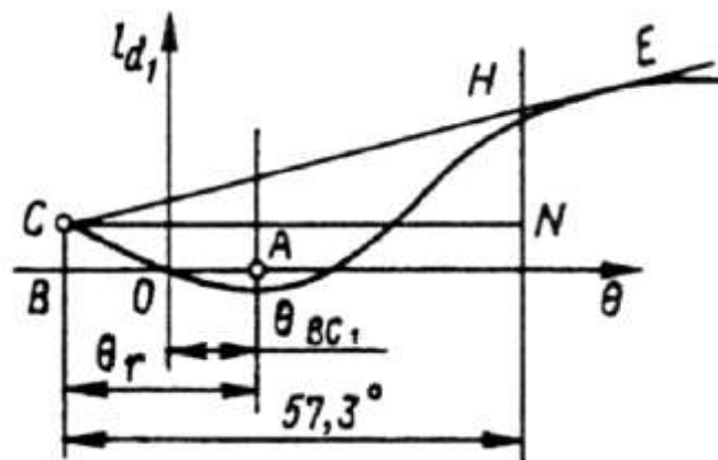
Рис. 3.1-1 Визначення перекидального моменту для днопоглиблювальних суден
