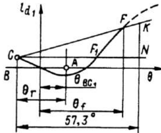
Рис. 3.1-2 Визначення перекидального моменту для днопоглиблювальних суден з урахуванням кута заливання
