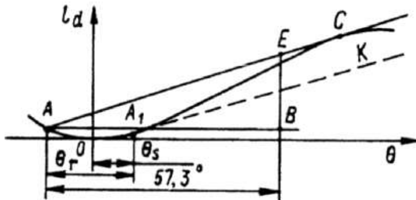
Рис.1.2.1 Визначення перекидального моменту плавучого крана при переході за діаграмою динамічної остійності
